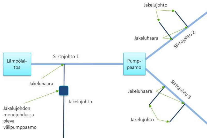
Kuva 11: Siirtojohto 1 haarautuu pumppaamossa siirtojohdoiksi 2 ja 3. Jakelujohtoon menojohtodossa oleva välipumppaamo on osa menojohtoa.
