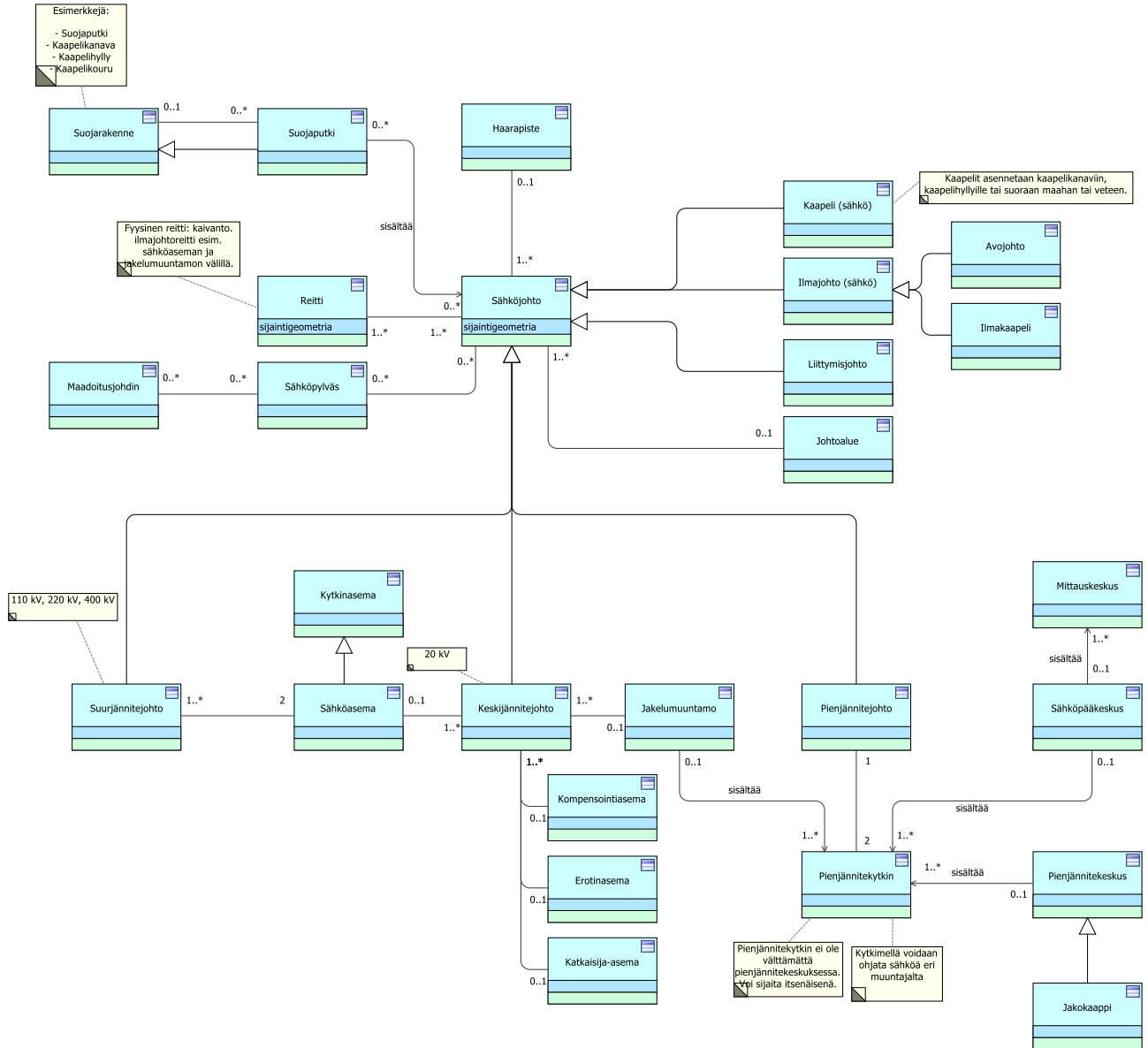
Kuva 4: Sähköverkko
